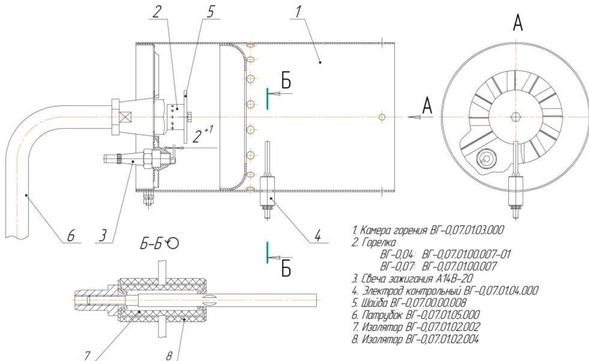
Рис.4 Камера горения воздушонагревателя ВГ-0,04, ВГ-0,07 в комплекте.
