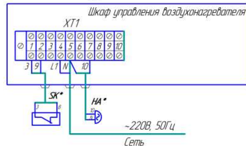
Рис.8 Схема электрическая соединений.
