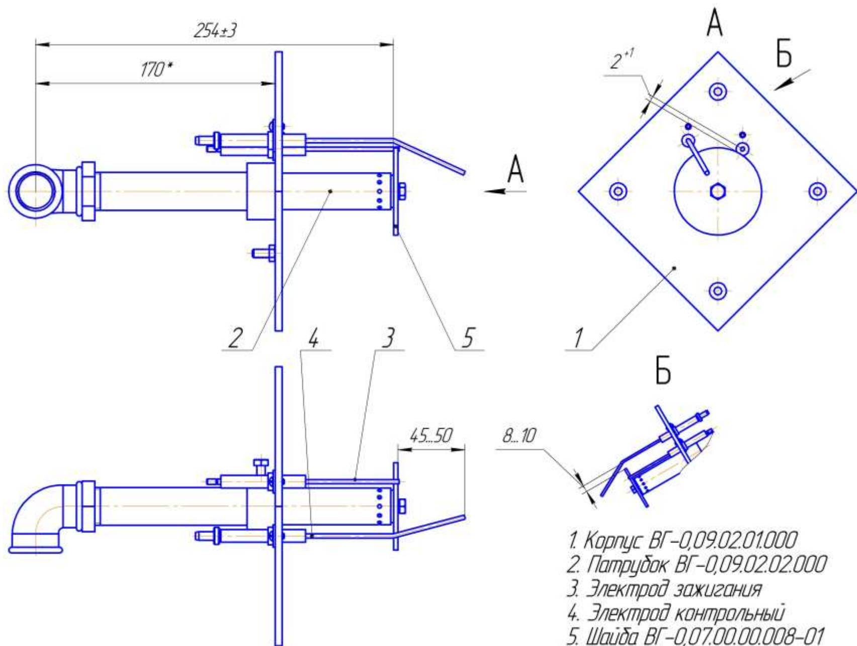
Рис.5 Горелка воздухонагревателя ВГ-0,09
