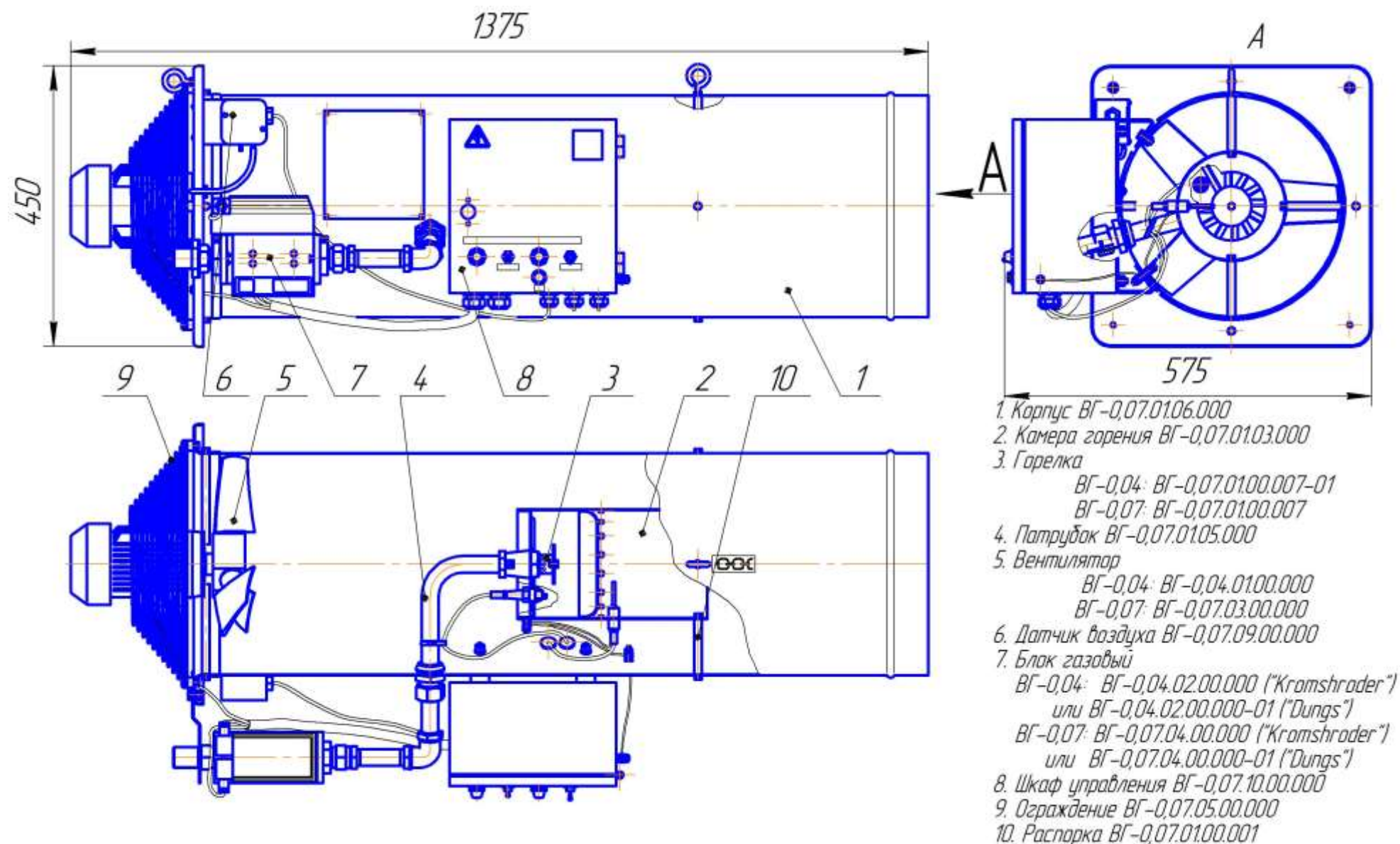
Рис.1 Воздухонагреватель газовый ВГ-0,04, ВГ-0,07.
