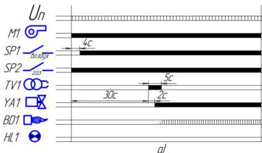
Диаграмма пуска при нормальном розжиге
