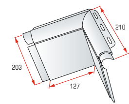
Угловой элемент откоса
