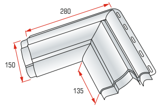
Угловой элемент наличника Модерн
