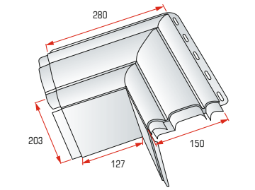
Угловой элемент «Наличник + откос» (в 2-х вариантах: «Классик»/«Модерн»)
