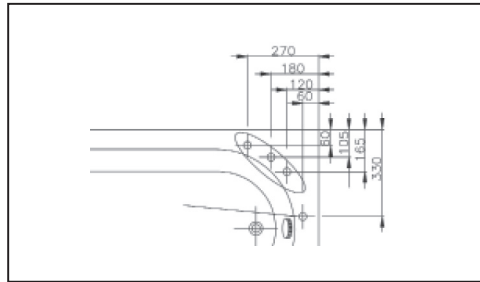
Bath Filler 4 Holes / Dört Delikli Batarya
