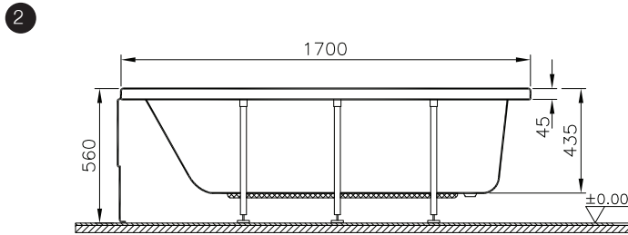
Front View Ön Görünüş
