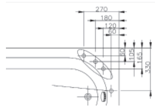
Bath Filler 4 Holes / Dört Delikli Batarya
