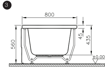
Side View Yan Görünüş
