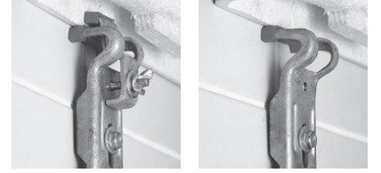
Detail A / Şekil A
