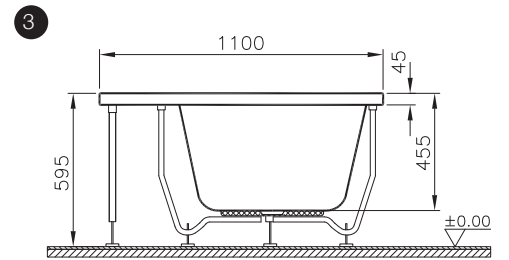
Side View Yan Görünüş
