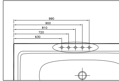
Bath Filler 5 Holes/Beş Delikli Batarya
