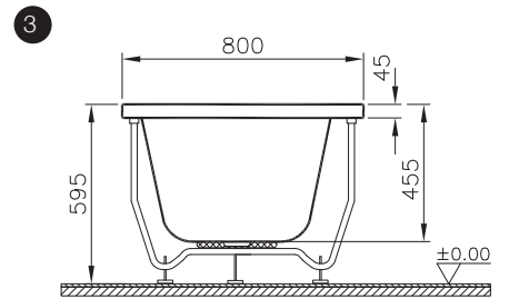
Side View Yan Görünüş
