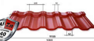
Металлочерепица "ЭТЕРНА" 350/25 мм
