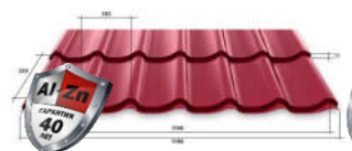
Металлочерепица "СУПЕР МОНТЕРЕЙ" 350/21 мм
