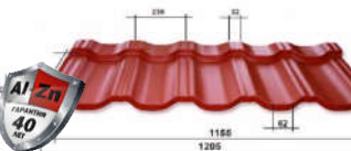
Металлочерепица "ЭТЕРНА ПЛЮС" 350/30 мм
