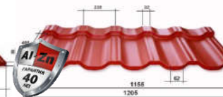
Металлочерепица "ВЕРОНА" 400/30мм
