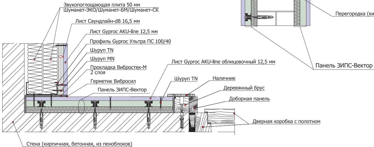
2.2.3 Угловое примыкание панелей ЗИПС-Вектор на стене к облицовке на каркасе 100 мм и дверному проему
