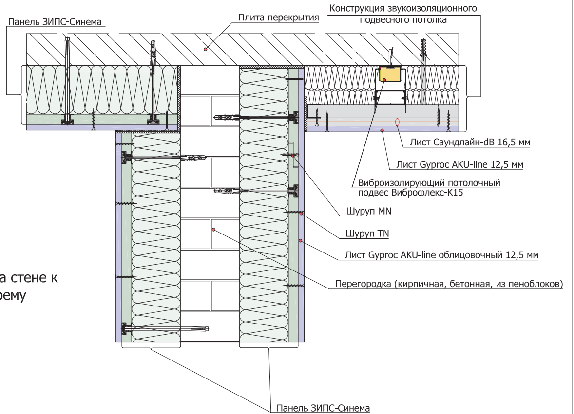
2.4.2 Примыкание панелей ЗИПС-Синема к панелям ЗИПС-Синема на потолочном перекрытии и подвесному звукоизолирующему потолку
